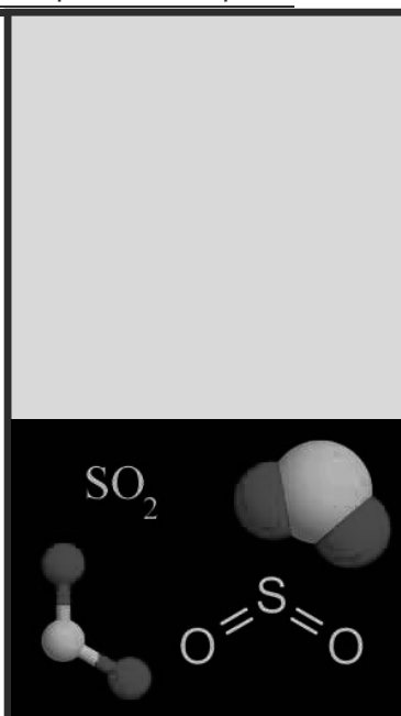
Слика бр. 51 Сумпор диоксид
