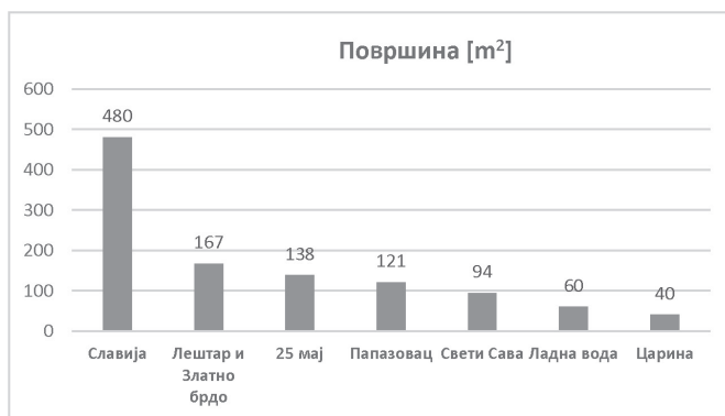
График 3.81 Површине објеката, у m²
