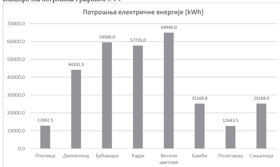
График 3.13 Потрошња електричне енергије објекта вртића, у kWh
