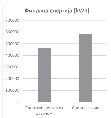
График 3.71 Финална енергија, у kWh
