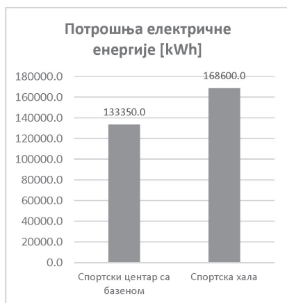
График 3.67 Потрошња електричне енергије објекта спорта, у kWh
