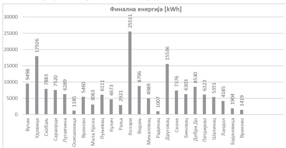
График 3.95 Финална енергија, у kWh
