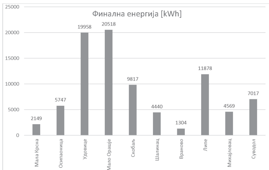
График 3.62 Финална енергија, у kWh
