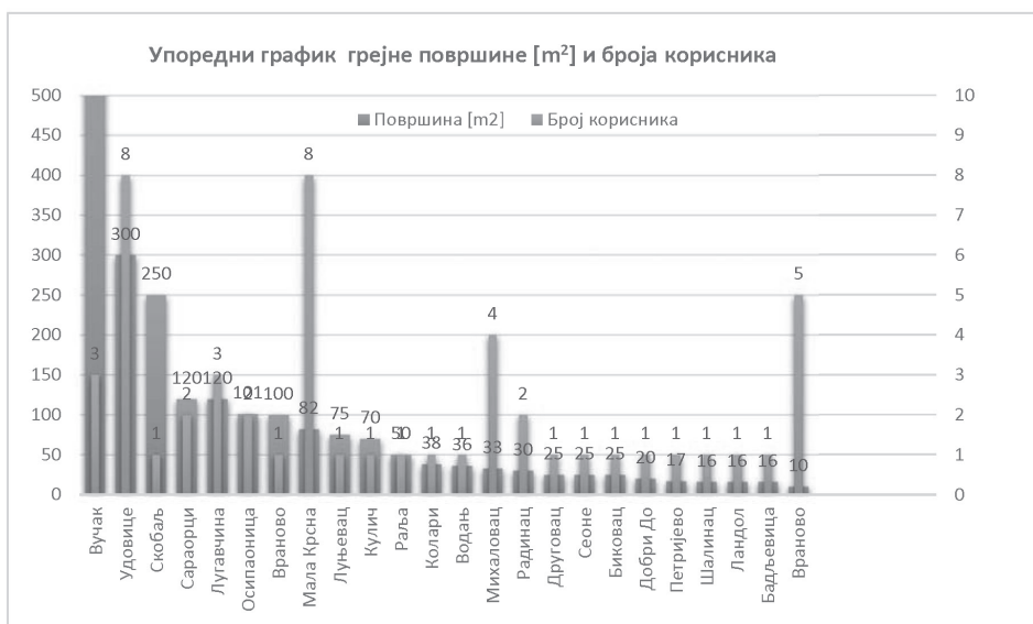
График 3.90 Упоредни график грејне површине објекта месних заједница и броја корисника
