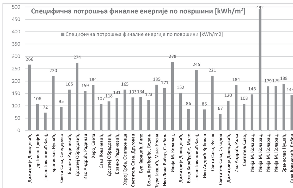
График 3.9 Специфична потрошња финалне енергије по површини, у kWh/m²
