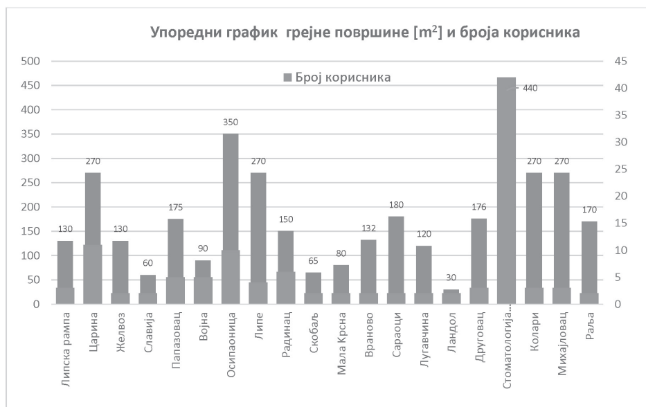
График 3.29 Упоредни график грејне површине објеката амбуланти и броја корисника
