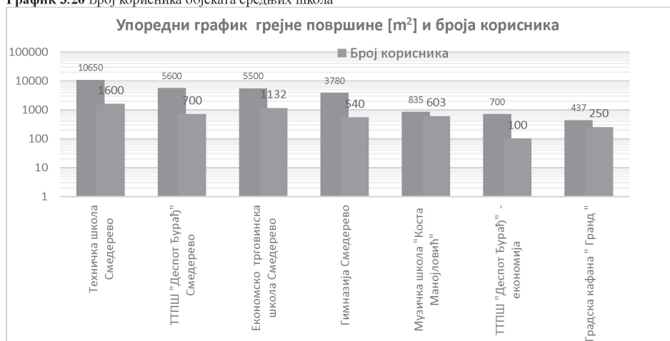
График 3.21 Упоредни график грејне површине објеката средњих школа и броја корисника
