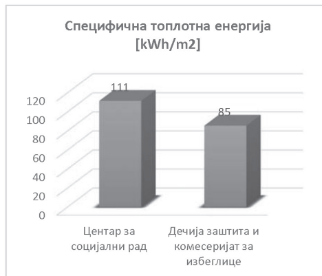
График 3.42 Специфична топлотна енергија, у kWh/m²
