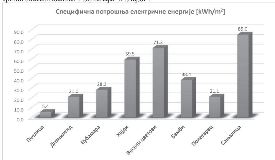
График 3.14 Специфична потрошња електричне енергије објекта вртића, у kWh/m 2
