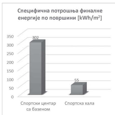
График 3.72 Специфична потрошња финалне енергије по површини, у kWh/m 2
